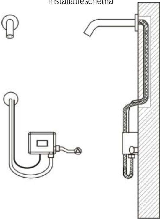
installatieschema
